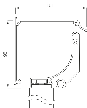
Flasque Type A
