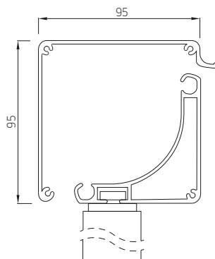
Flasque Typ C
